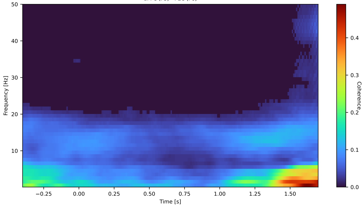
dPFC (F3) - PEC (P8)
